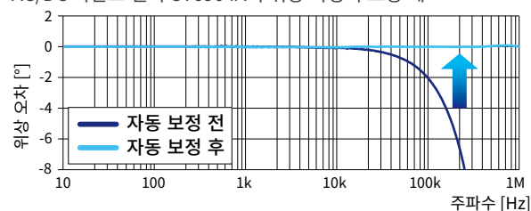
AC/DC 커런트 센서 CT6904A의 위상 특성의 보정 예
